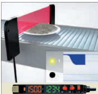
Два выхода усилителя E3X-DA-S можно использовать для распознавания двух отличающихся уровней яркости.
