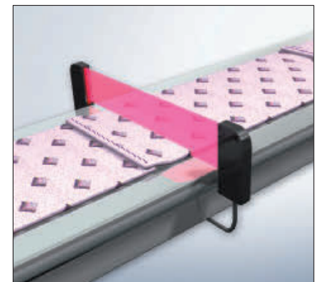
Срабатывание по одному или двум фронтам сигнала
