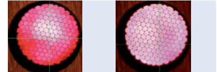
Распределение света в многоволоконном кабеле с обычными усилителями Распределение света в усилителе E3X-DA-S нового поколения
